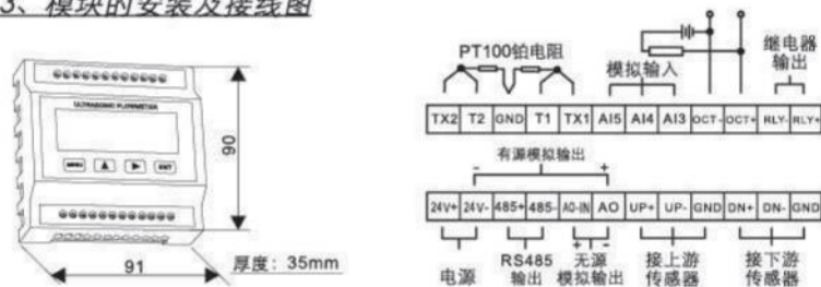
安装图
