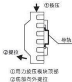
拆卸图
