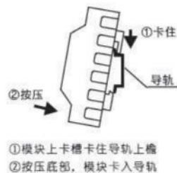
安装图
